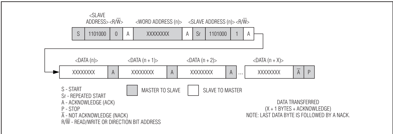
图5. 写/读数据(写指针，然后是读指针)——从设备的接收和发送
